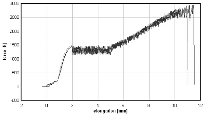
Rys. 3. Wyniki trzech testów rozciągania próbki ze stali nierdzewnej przeprowadzonych w temperaturze ciekłego helu [10]
